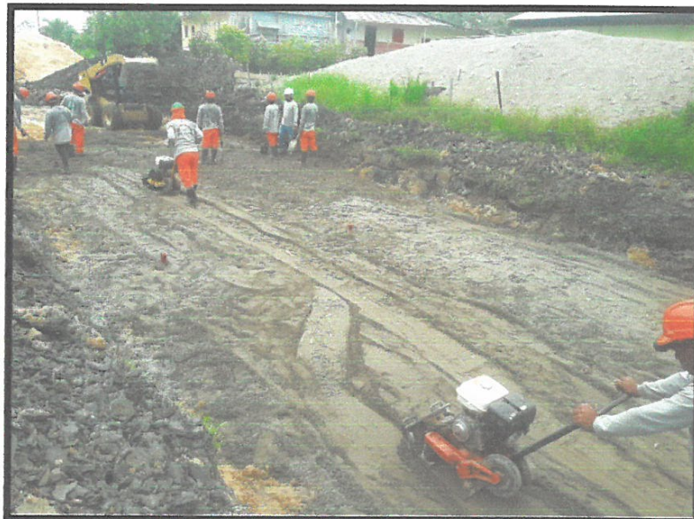
SUBRASANTE MEJORADA CON MATERIAL DE PRESTAMO 0+280
