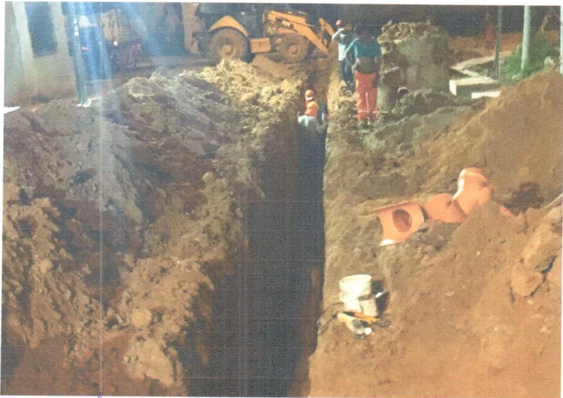
INSTALACION DE LA TUBERIA DE DESAGUE.
