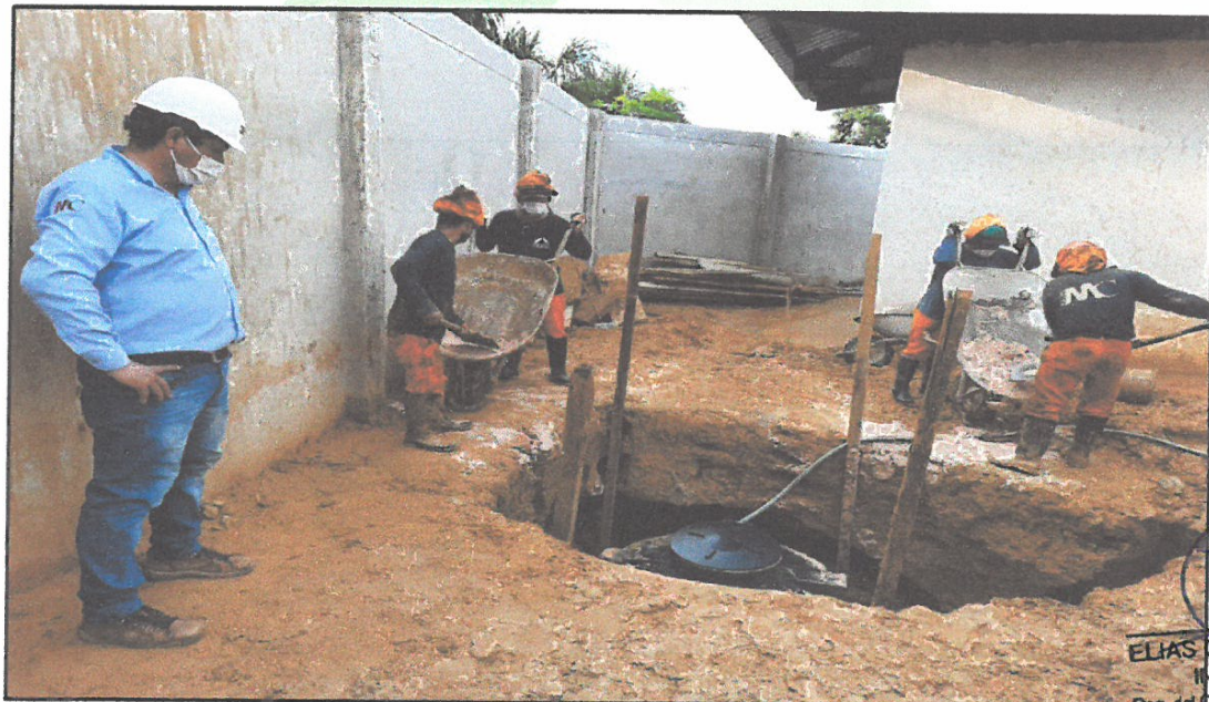
FOTO N°04: VISTA DE INSTALACIÓN DE TANQUE BIODIGESTOR.
