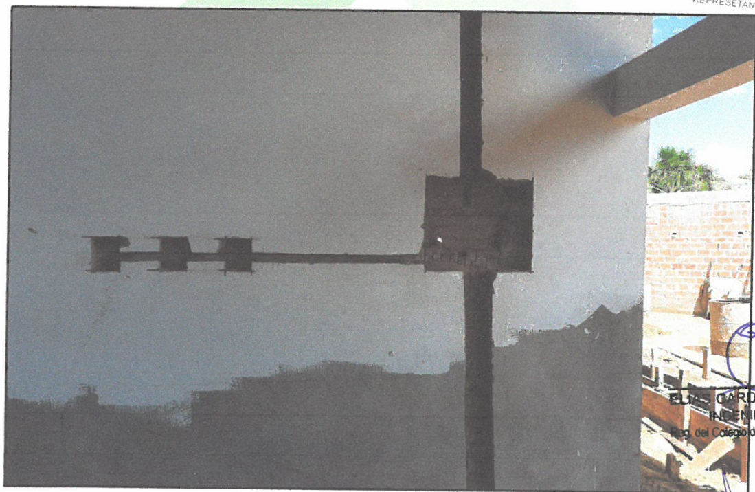
FOTO N° 14: PICADO DE PARED PARA COLOCACIÓN DE CONDUCTORES EN INSTALACIONES ELECTRICAS PARA SALIDAS DE TOMACORRIENTES Y INTERRUPTORES Y TABLEROS
