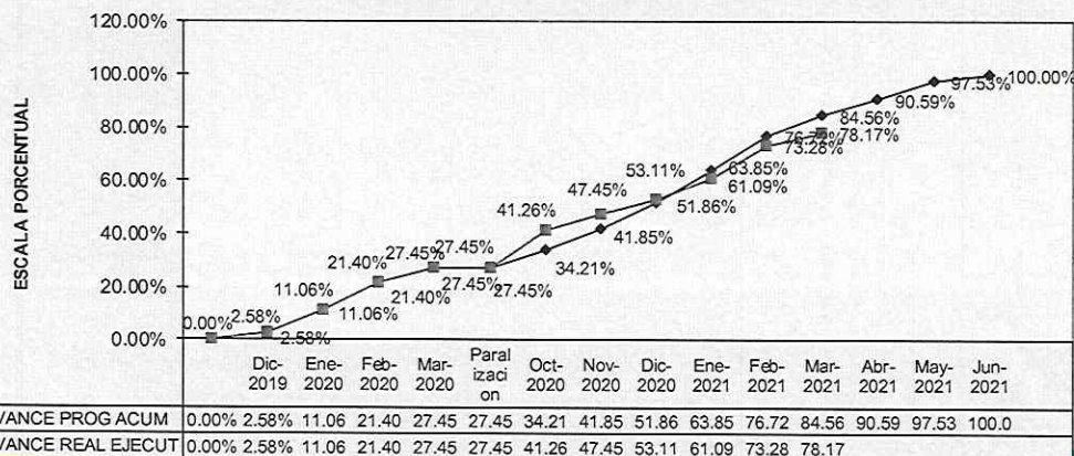
CURVA DE CONTROL DE AVANCE FÍSICO
